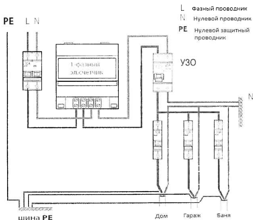
Пример выполнения трехпроводной сети для подключения 1 фазных потребителей.
